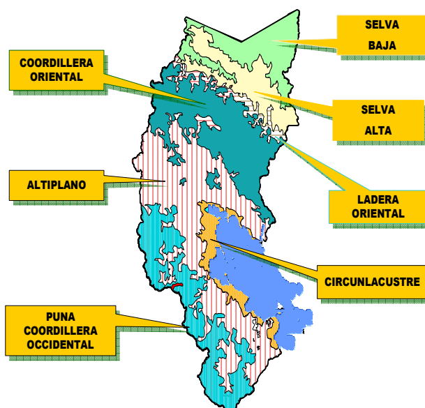
MAPA DE PISOS ECOLÓGICOS DE LA REGIÓN PUNO
